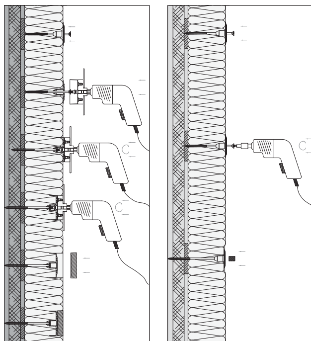
Montaj ascuns conf. principiului STR, cu rondelă STR
